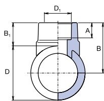
Вварное седло
