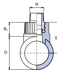
Вварное седло
