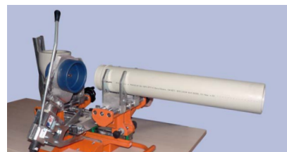
перемещение после нагрева
